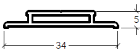
Seuil plat
