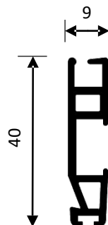
BARRE DE CHARGE CRIQUET/PIED REGLABLE
